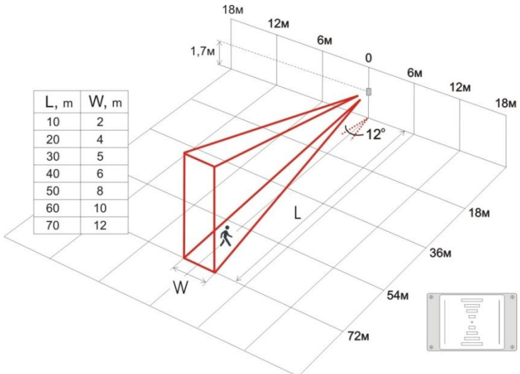
Рис. 6 Размер зоны при горизонтальной установке датчика на стене внутри помещения
