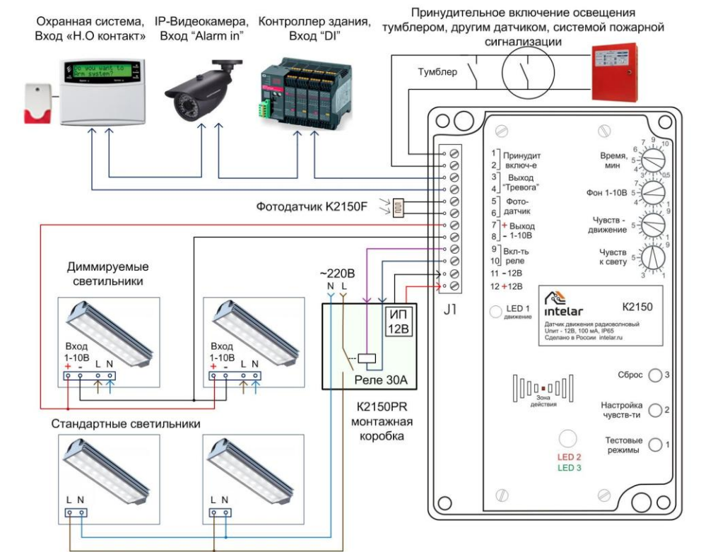
Рис. 1 Схема, поясняющая принцип соединения датчика K2150 с внешними устройствами. Не является монтажной схемой! Монтажная схема – см. стр. 4.
