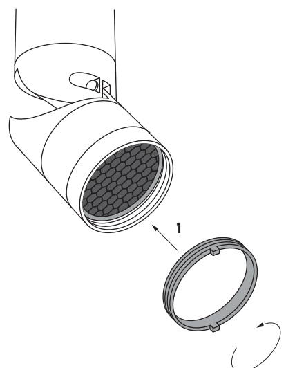
Закрутить прижимное кольцо
